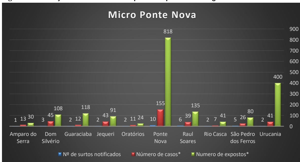
Figura 3. Distribuição de surtos notificados por município na microrregião de Ponte Nova
